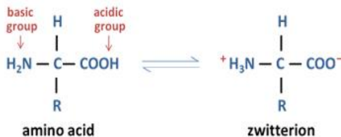
Fig. 12: Zwitterion
