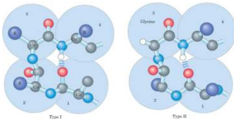
Fig. 7: \beta -Turns
