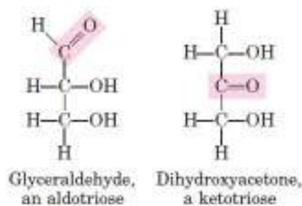
Fig. 2: Trioses
