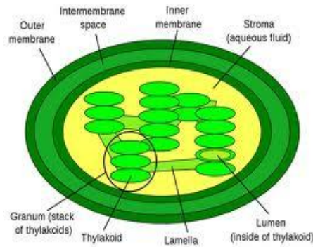
Fig. 9: Chloroplast
