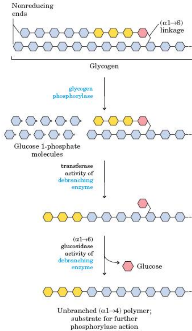
Fig. 5 Glycogenolysis
