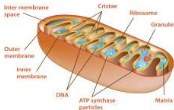
Fig. 8: Mitochondria
