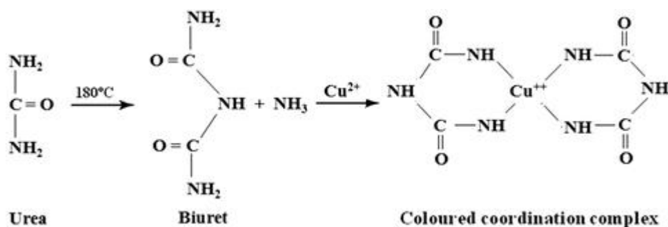
Fig. 10 Biuret reaction
