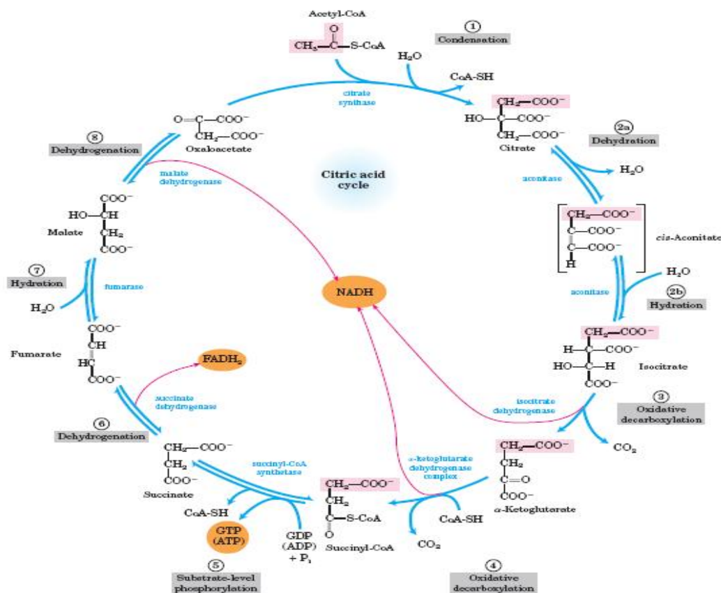
Fig. 9 TCA cycle
