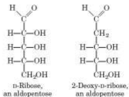
Fig. 3: Pentoses
