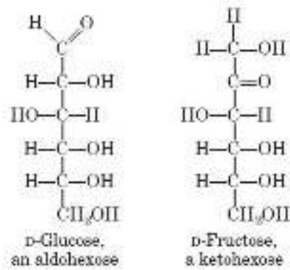
Fig. 4: Hexoses
