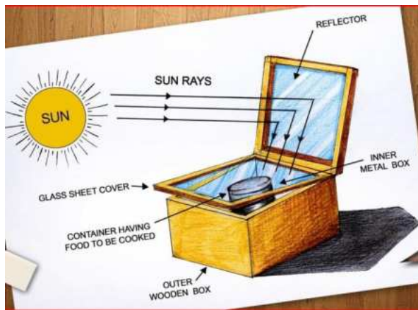
Fig. 3. Solar cooker
