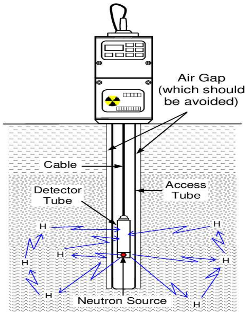
Fig.4 Neutron moisture meter
